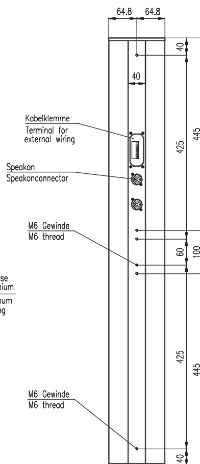
Rückansicht
