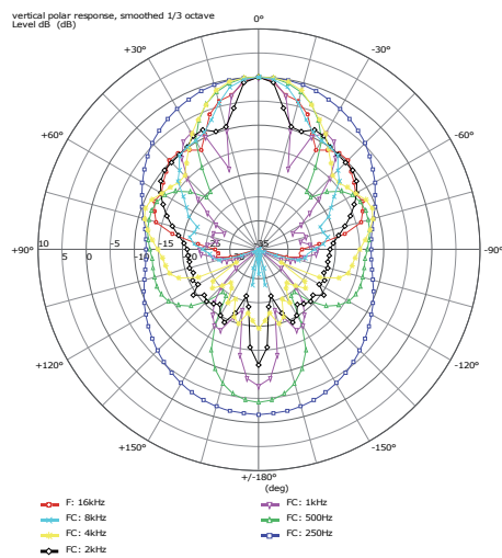
Bild 3: Polardiagramm vertikal
