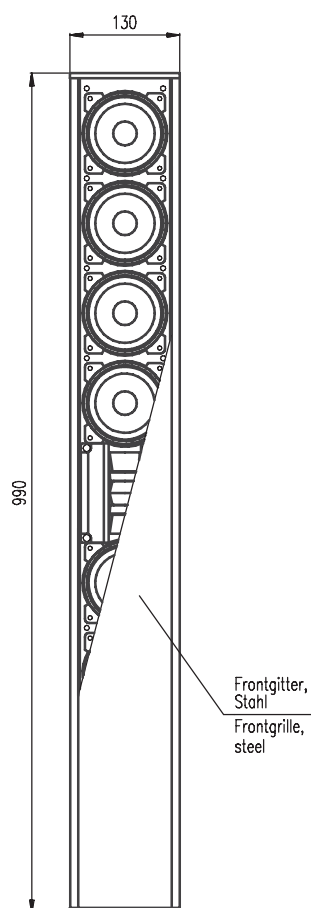
Vorderansicht
