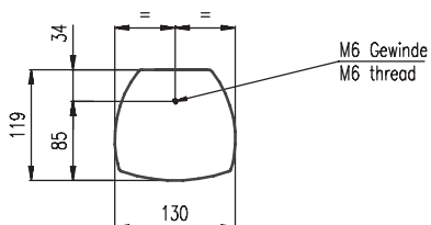
Draufsicht
