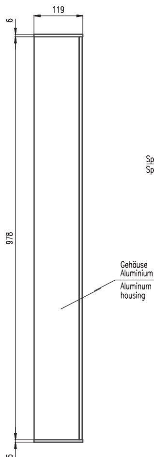
Seitenansicht
